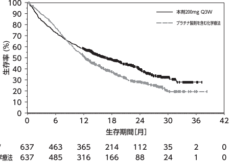
図11 OSのKaplan-Meier曲線（KEYNOTE-042試験） （PD-L1発現がTPS≥1%の患者）
