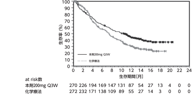
図15 OSのKaplan-Meier曲線（KEYNOTE-045試験）
