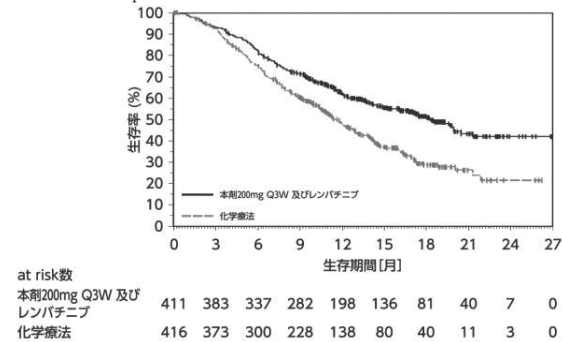
図28 OSのKaplan-Meier曲線 (KEYNOTE-775/E7080-309試験)
