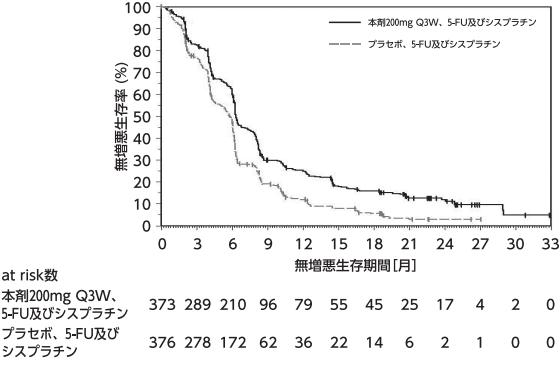
図23 PFSのKaplan-Meier曲線（KEYNOTE-590試験）
