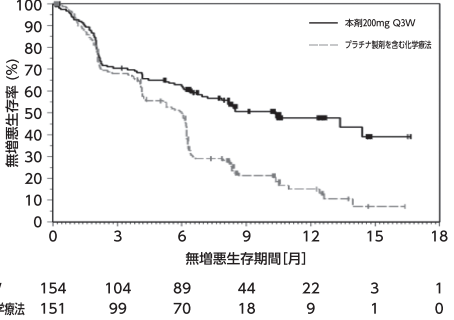
図12 PFSのKaplan-Meier曲線（KEYNOTE-024試験） （PD-L1発現がTPS≥50%の患者）
