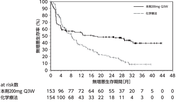
図25 PFSのKaplan-Meier曲線（KEYNOTE-177試験）
