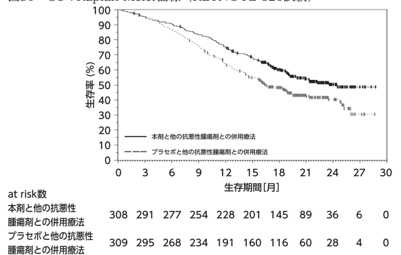
図30 OSのKaplan-Meier曲線 (KEYNOTE-826試験)
