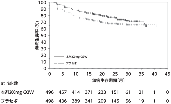
図19 DFSのKaplan-Meier曲線 (KEYNOTE-564試験)
