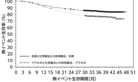
図27 EFSのKaplan-Meier曲線（KEYNOTE-522試験）
