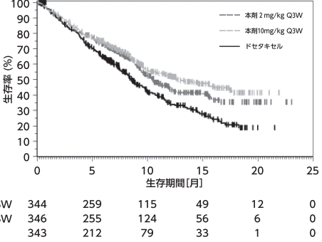
図14 OSのKaplan-Meier曲線（KEYNOTE-010試験） （PD-L1発現がTPS≥1%の患者）
