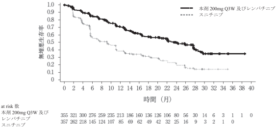
図18 PFSのKaplan-Meier曲線 (E7080-307/KEYNOTE-581試験)
