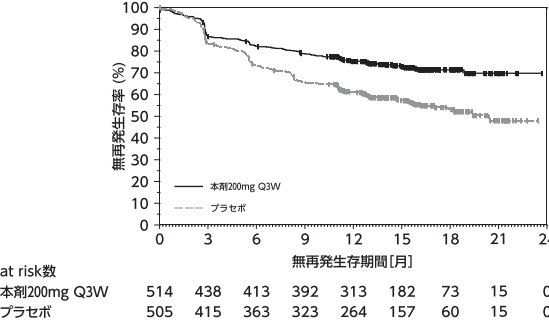
図5 RFSのKaplan-Meier曲線 (EORTC-1325-MG/KEYNOTE-054試験)
