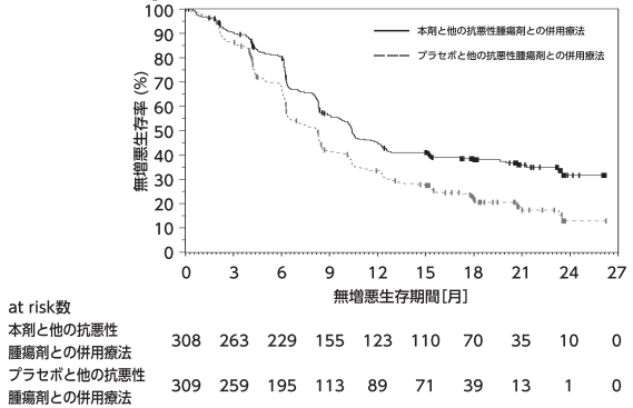
図31 PFSのKaplan-Meier曲線（KEYNOTE-826試験）
